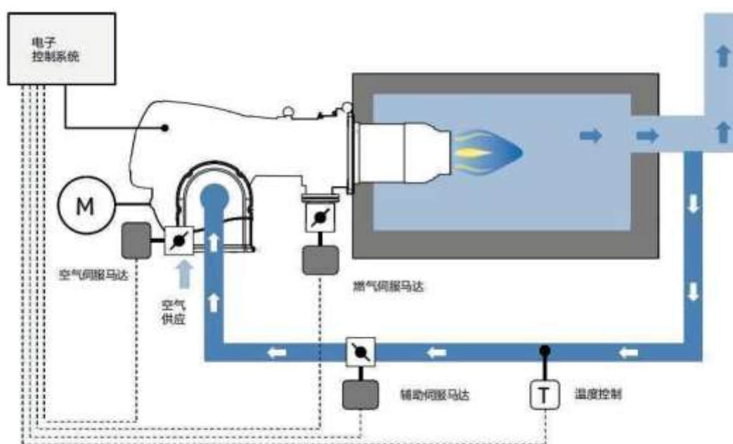
低氮燃燒器技術示意圖
