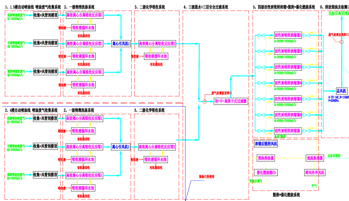
廢氣處理工藝流程
