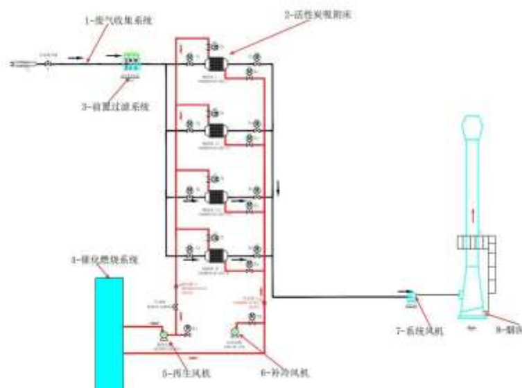
廢氣處理工藝流程
