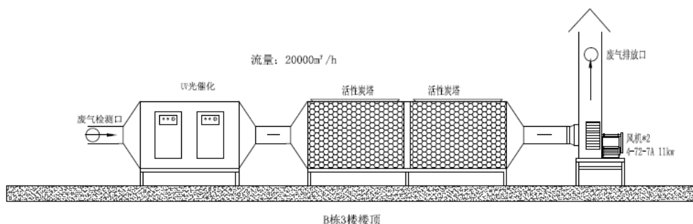
紫外線光催化及活性炭吸附流程圖
