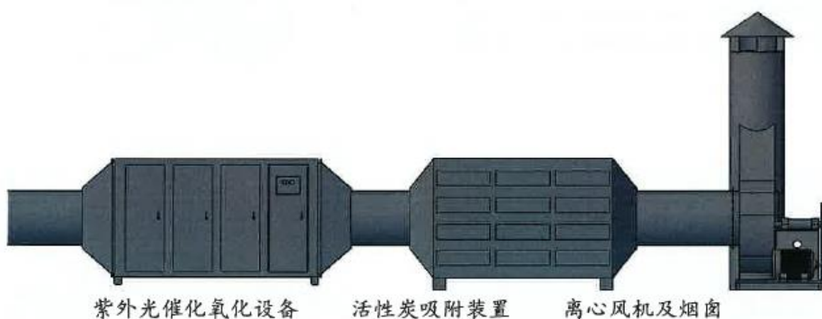
紫外線光催化及活性炭吸附流程圖
