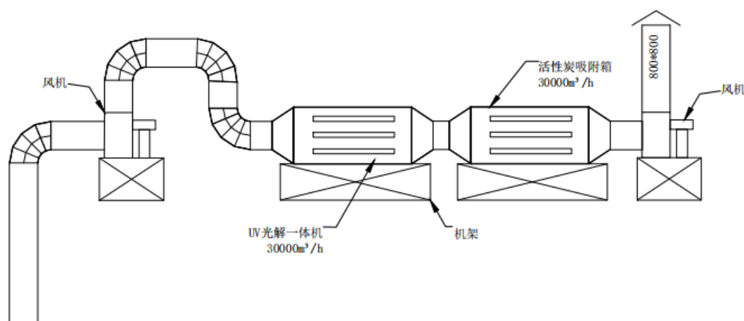
紫外線光解及活性炭吸附流程圖
