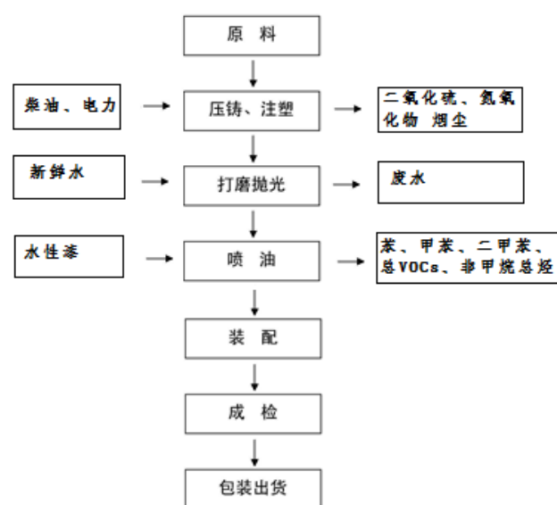
生產流程圖
