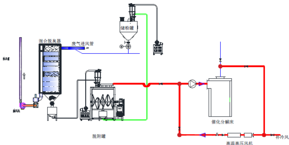
工藝流程圖
