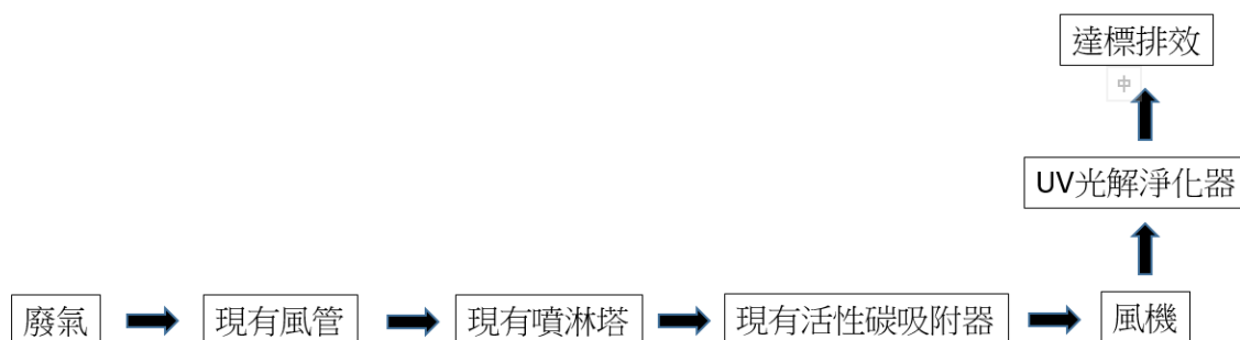
有機廢氣淨化系統（噴淋、活性炭、UV 光解）的工藝流程圖
