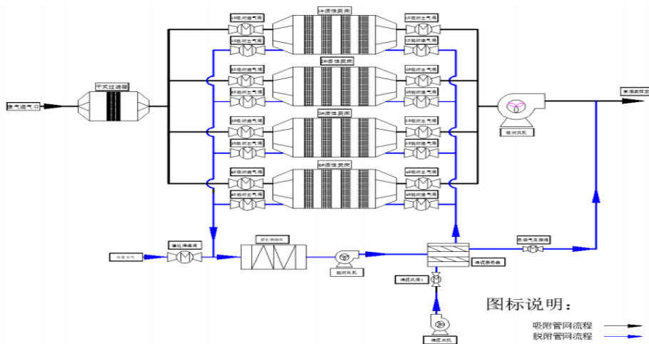
工艺流程图
