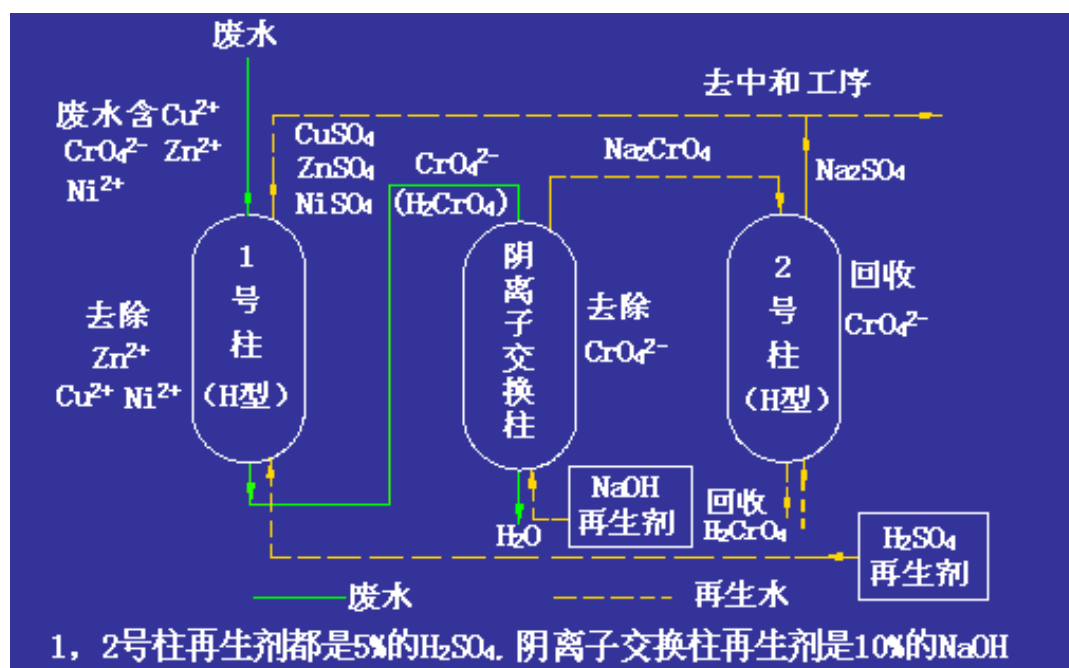
「電鍍廢水離子交換回用系統」技術簡介
